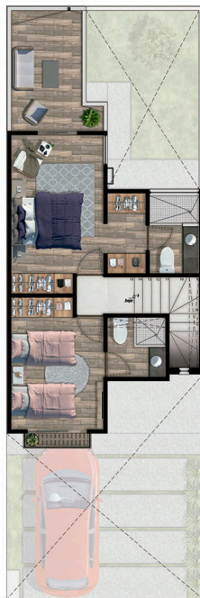
PLANTA ALTA
